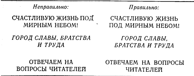
Рис. 17.14. Двухстрочные заголовки
