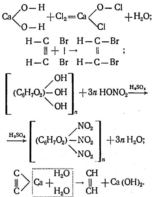
Рис. 12.51. Структурные формулы
